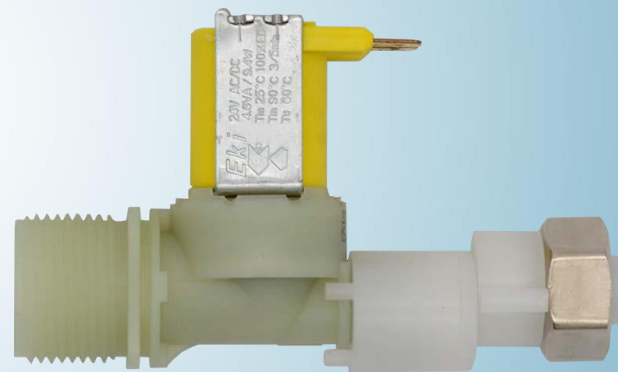
Elektromagnetni ventil 0402
