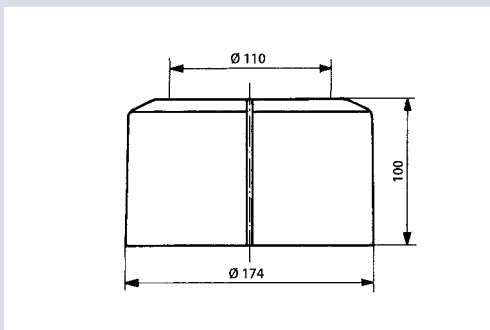
Pokrivna rozeta DN100
