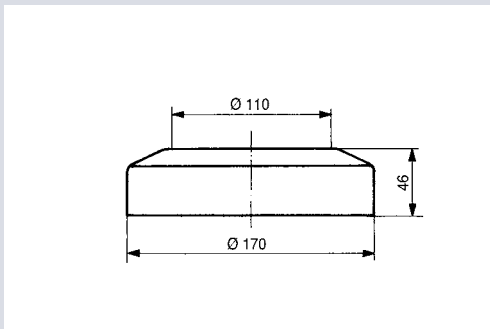
Ravna rozeta DN100
