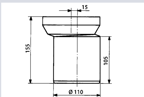
Izmični nastavak DN100
