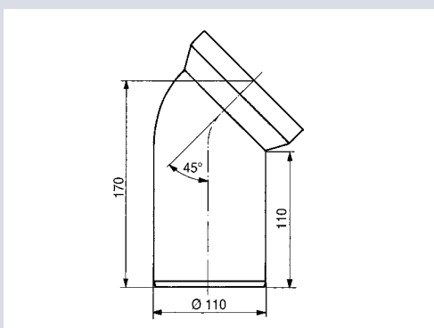
Priključno koljeno za WC od 45° DN100
