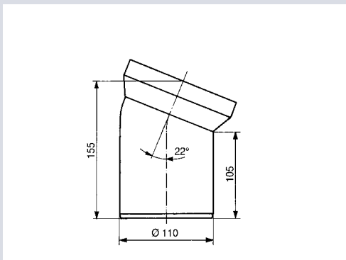
Priključno koljeno za WC od 22° DN100
