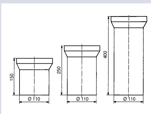
Priključni nastavak za WC DN100
