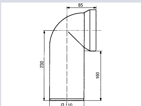
Priključno koljeno za WC od 90° DN100
