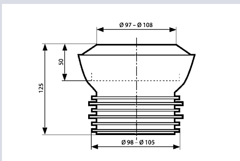
Manšeta (objumica) za WC
